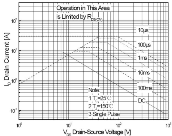
图 6 最大安全工作区曲线 Fig6 Maximum Safe Operating Area
