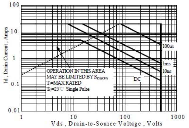
图 9 最大安全工作区曲线
