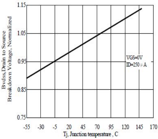
图 3 击穿电压与温度曲线
