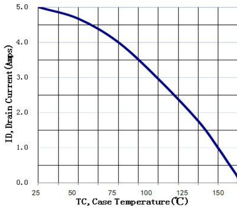
图 8 最大漏极电流与壳温曲线
