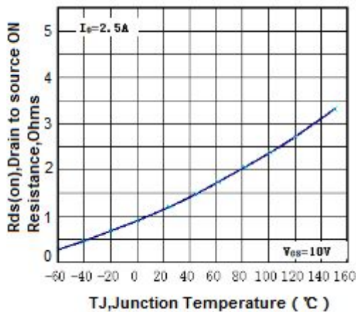
图 5 导通电阻与温度曲线
