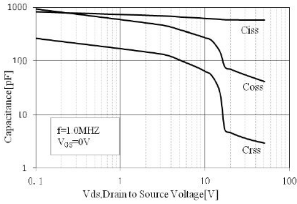
图 6 电容与漏源电压曲线
