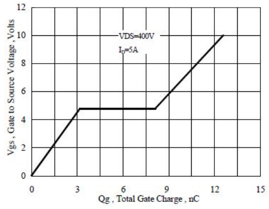
图 7 栅极电荷与栅源电压曲线
