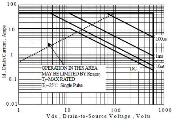
图 6-1 SIF12N60F(TO-220)
