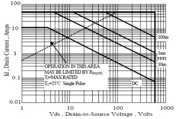
图 6-2 SIF12N60F(TO-220FP(L))
