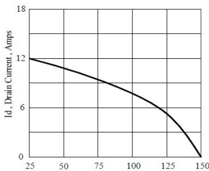
图 5 最大漏极电流与壳温曲线
