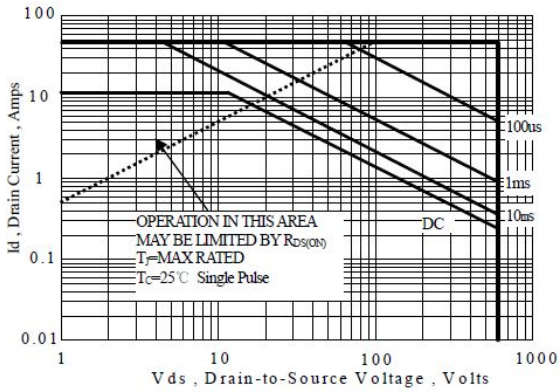
图 6-3 SIF12N60F(TO-262&263)
