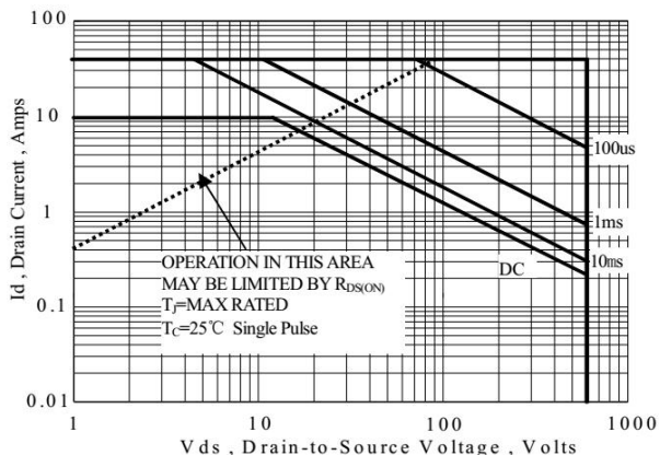
图 6-1 SIF10N60F(TO-220)
