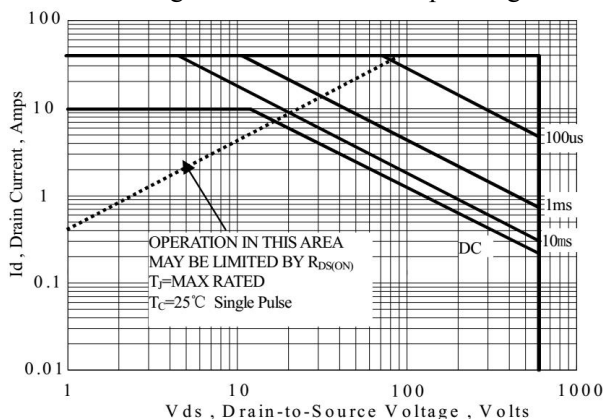
图 6-3 SIF10N60F(TO-262&263)
